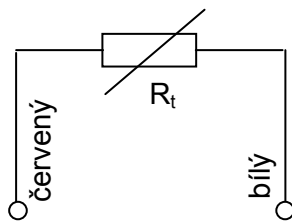
dvouvodičové
